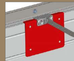
PLAQUE RENFORT ACCROCHE MOTEUR
