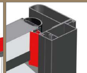
JOINT TUBULAIRE À LÈVRES CÔTÉ FERMETURE
