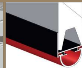
JOINT INFÉRIEUR CAOUTCHOUC
