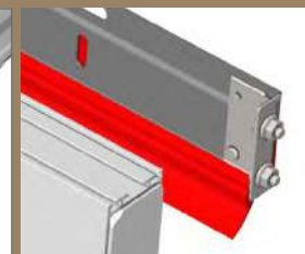
PROFIL LINTEAU AVEC JOINT EPDM
