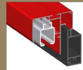
PRÉCADRE NOIR AVEC PROFIL DE RAIL MONOBLOC
