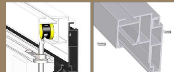
CHARIOT 4 ROULETTES SUR ROULEMENT AXE EN INOX
