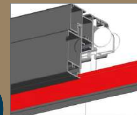
JOINT D'ÉTANCHÉITÉ EPDM SUR LINTEAU
